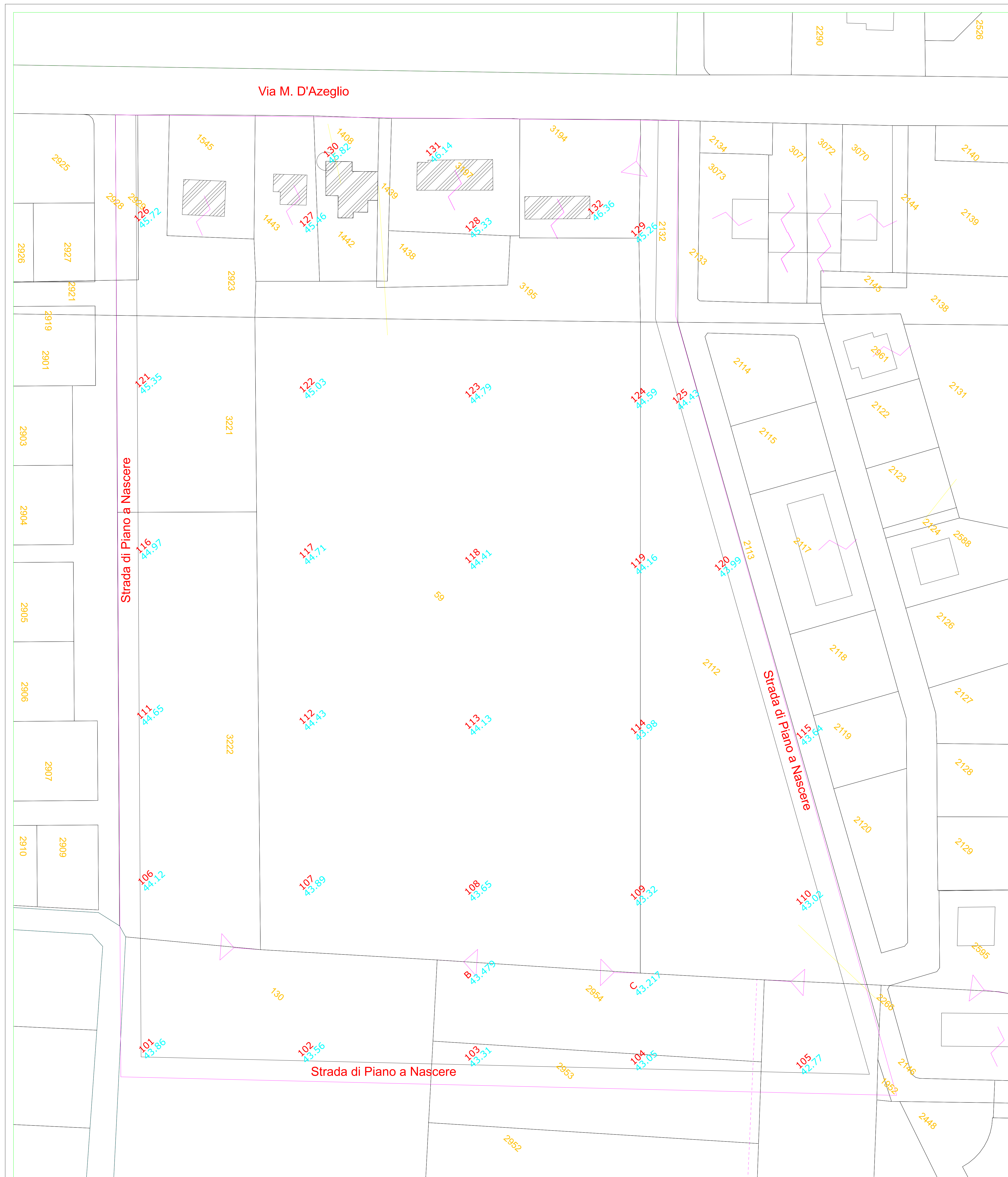
RILIEVO PLANOALTIMETRICO SU BASE CATASTALE
