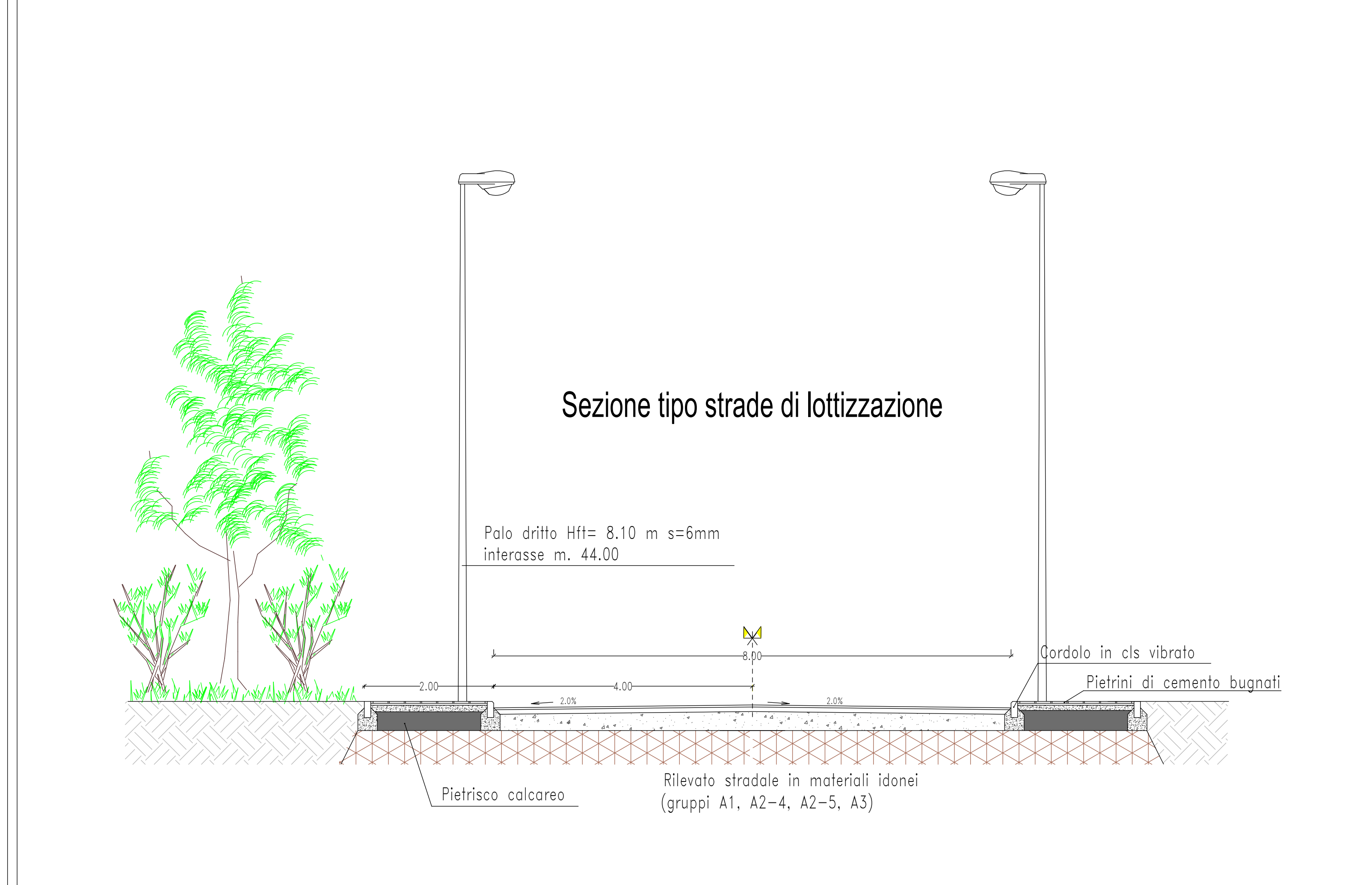
SEZIONI STRADALI TIPO E PARTICOLARI COSTRUTTIVI
